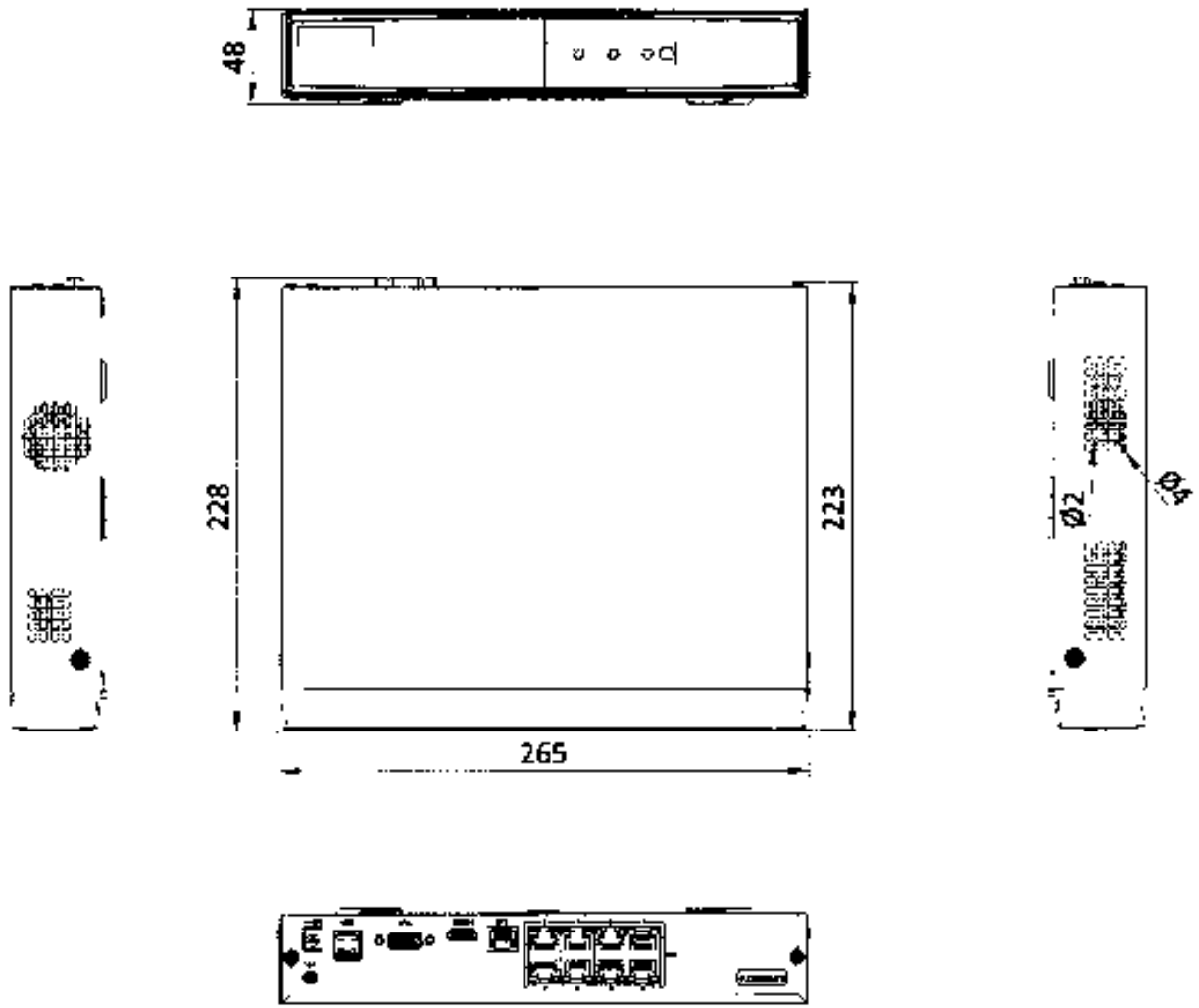
scale/1:1;Unit/mm
